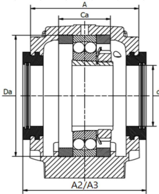
Labyrinth A2 / Taconite A3
