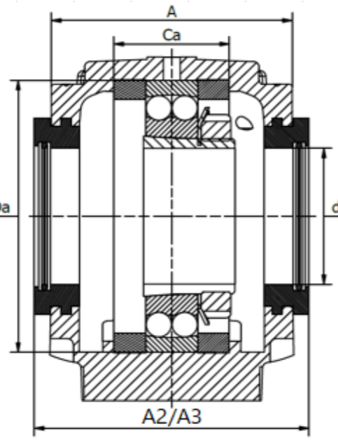
Labyrinth A2 / Taconite A3
