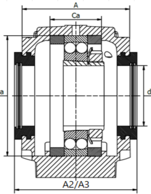
Labyrinth A2 / Taconite A3
